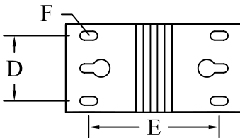
VUE DE DESSOUS / BOTTOM VIEW TYPE FERMÉ / CLOSED TYPE
