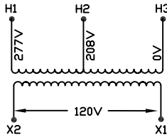
DIAGRAMME DE CONNEXION / CONNECTION DIAGRAM
