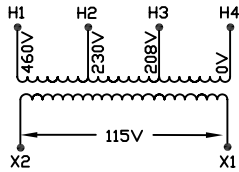
DIAGRAMME DE CONNEXION / CONNECTION DIAGRAM
