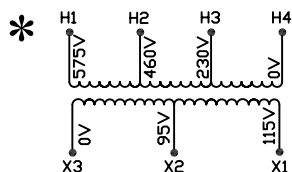
DIAGRAMME DE CONNEXION / CONNECTION DIAGRAM
