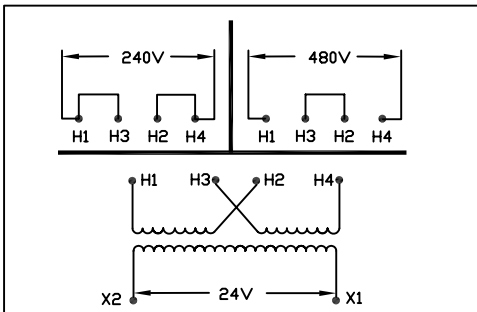
DIAGRAMME DE CONNEXION/ CONNECTION DIAGRAM
